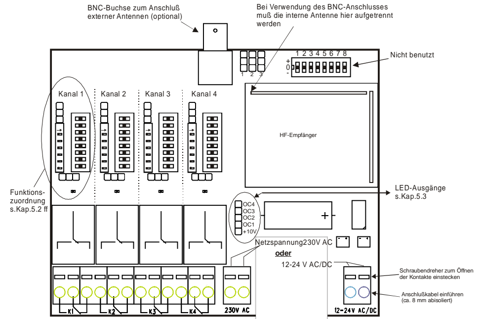
Bild 1: Funktionsübersicht SHR-12 K4
