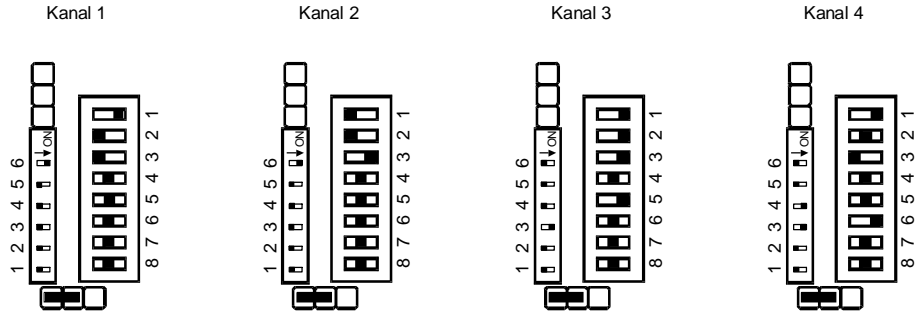
Bild 4: Beispiel einer Kombination von Befehlen am Auswahlfeld des SHR-12 K4
