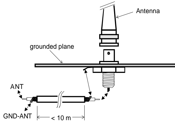
Bild 1: Anschluss eines Antennenkabels Fig. 1: Connection of an antenna cable Schéma 1: Connexion du câble de l'antenne
