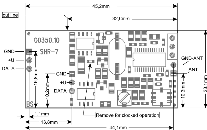
Image 1 : module-récepteur et schéma des connexions.
