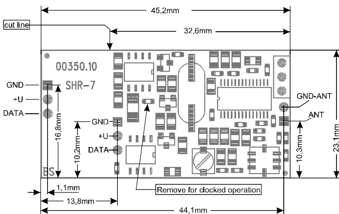
Bild 1: Empfangsmodul SHR-7 mit Anschlussbelegung
