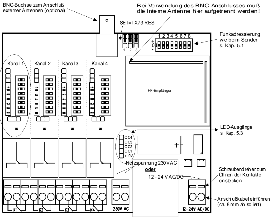
Bild 1: Funktionsübersicht Empfänger
