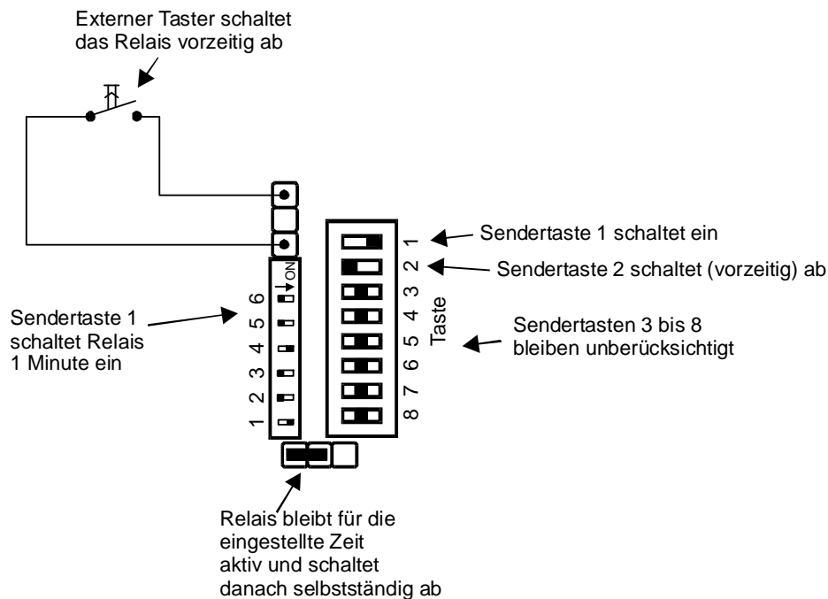
Bild 3: Beispiel einer Befehlszuordnung mit Handsendern am Auswahlfeld des Empfängers
